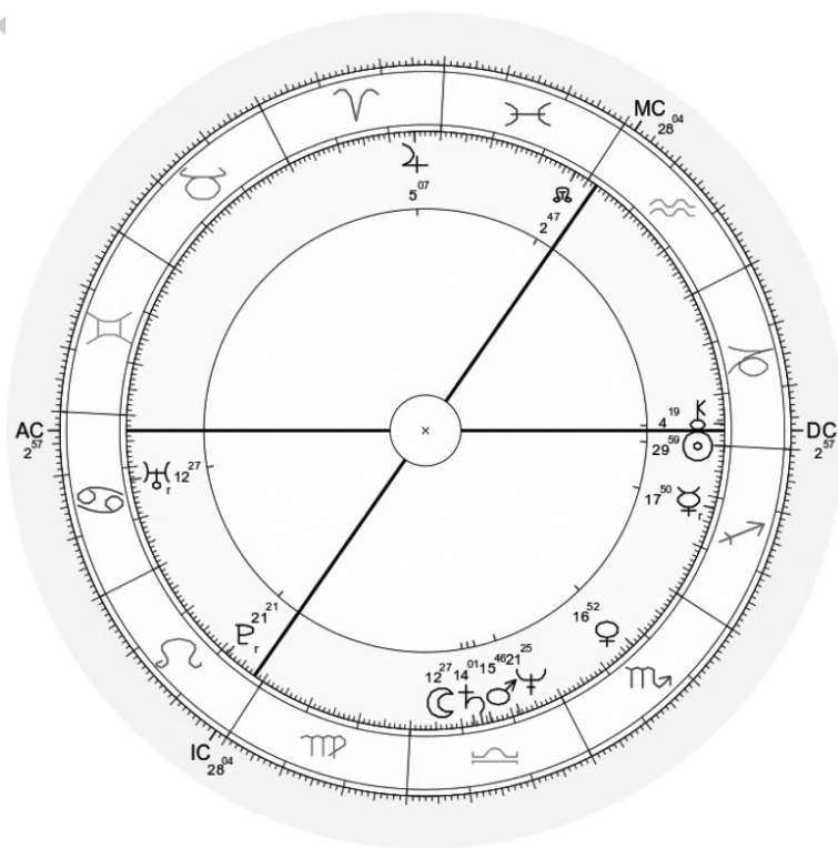
星圖一・1951年12月22日的倫敦冬至圖
