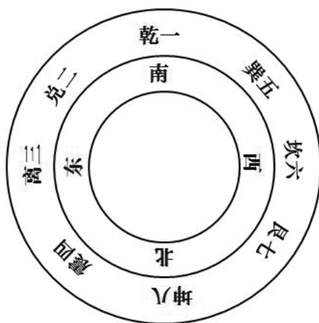
先天八卦圖
